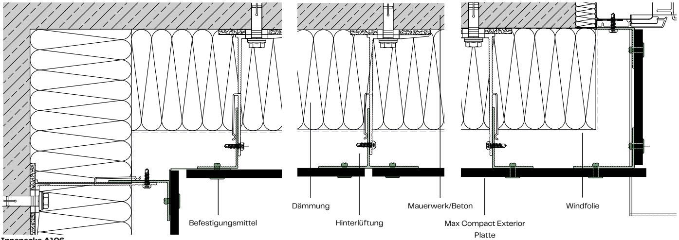
Innenecke A106
