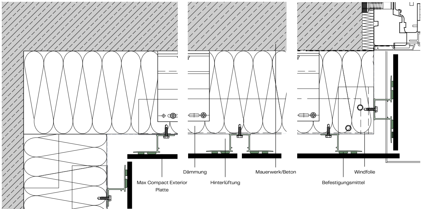
Innenecke A106
