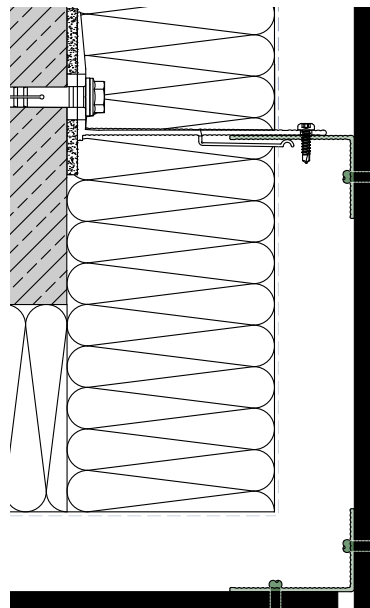
Außenecke A105
