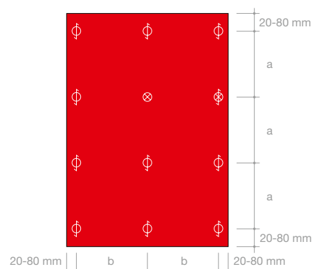
TRAMO DOBLE Fig. 39
