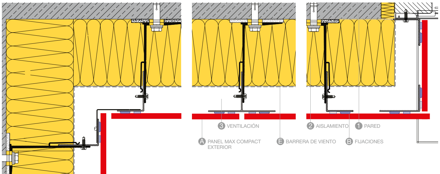
ESQUINA INTERIOR A106
