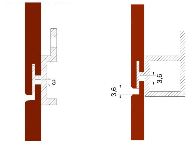
Figura 4.1a: Junta horizontal con grapa y perfil continuo.
