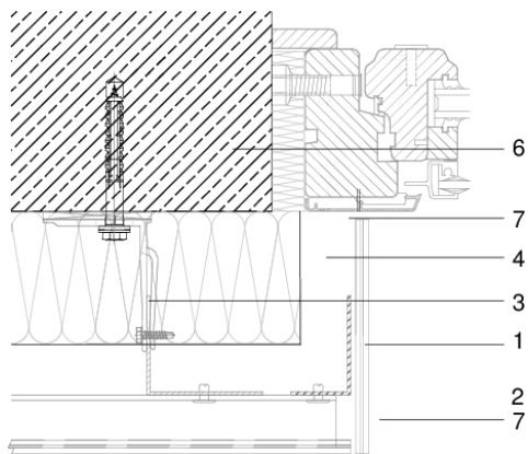
Figura 5.9b: Sección horizontal con perfil continuo. Telar de jamba con perfil auxiliar.
