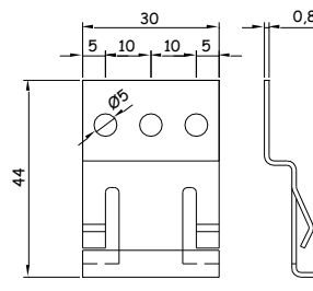
3. Potdekselklem
