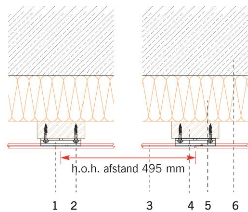
Horizontale doorsnede
