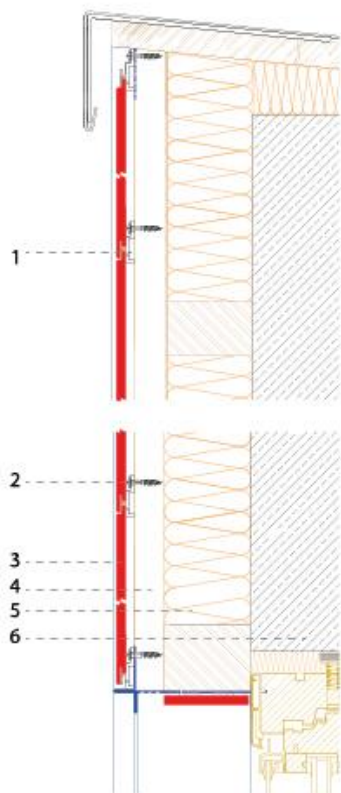
Verticale doorsnede
